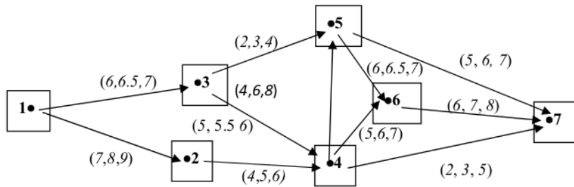
Gambar 5.4.1. Suatu Jaringan Berkapasitas Fuzzy
