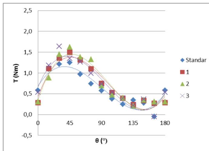
Gambar 3. Hubungan Torsi statik dengan posisi sudu pada panjang plat pengarah 105 mm
