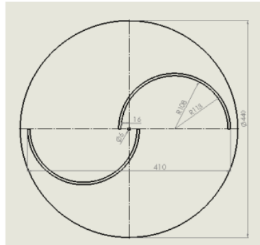
Gambar 1. Dimensi kincir angin Savonius
