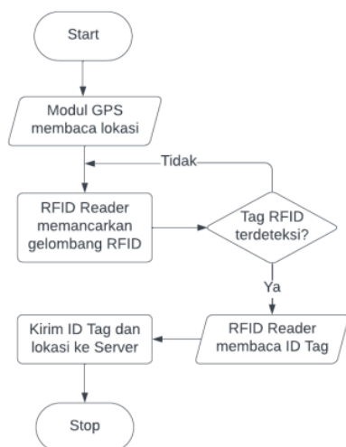
Gambar 5. Flowchart cara kerja alat penghitung kecepatan terbang merpati pos pada prototipe
