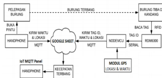
Gambar 4. Diagram blok cara kerja alat penghitung kecepatan terbang merpati pos
