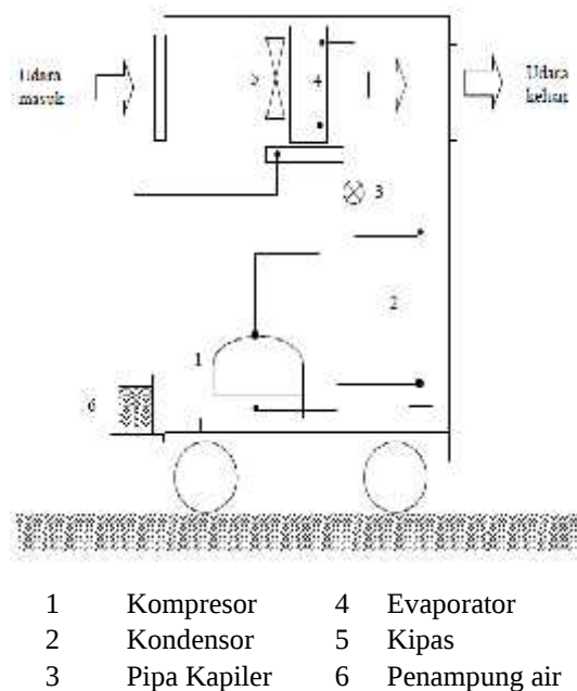
Gambar 3 Skematik penyejuk udara Siklus kompresi uap
