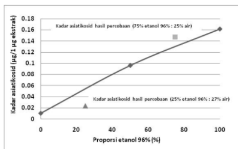
Gambar 1. Respon proporsi etanol vs kadar asiaticosid hasil maserasi pada suhu 50°C dengan persamaan Y = 0,1617 (X_1) + 0,0104 (X_2) + 0,0408 (X_1)(X_2)
