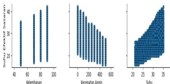
Gambar 4. Plot Hubungan Variabel Prediktor dengan Variabel Respon
