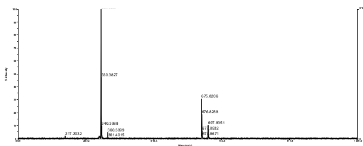
Gambar 2. Spektra massa dari senyawa hasil sintesis
