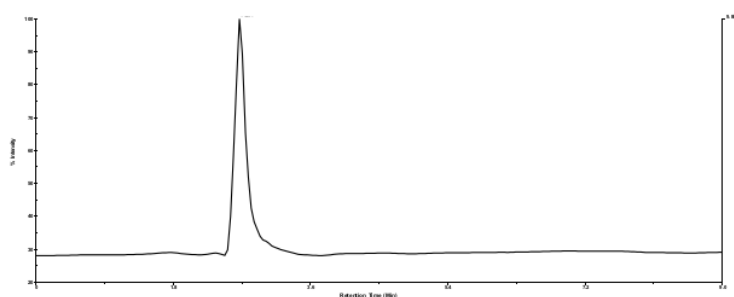
Gambar 1. Kromatogram LC senyawa hasil sintesis
