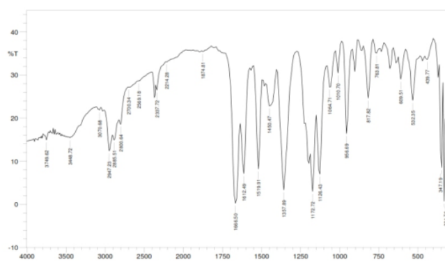
Gambar 3. Spektrogram infra merah senyawa hasil sintesis
