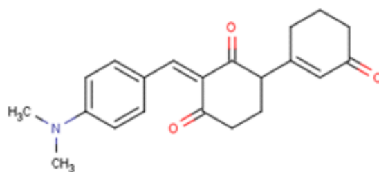
Gambar 5. Struktur senyawa 2-(4-(dimetilamino)benzilidena)-4-(3-oksosiklohex-1-enil) sikloheksana-1,3-dion
