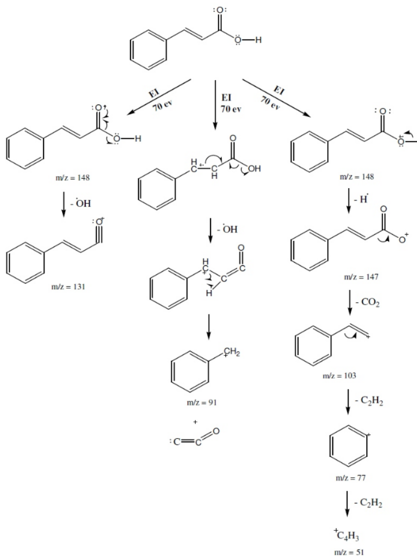
Gambar 5. Usulan mekanisme fragmentasi senyawa hasil sintesis
