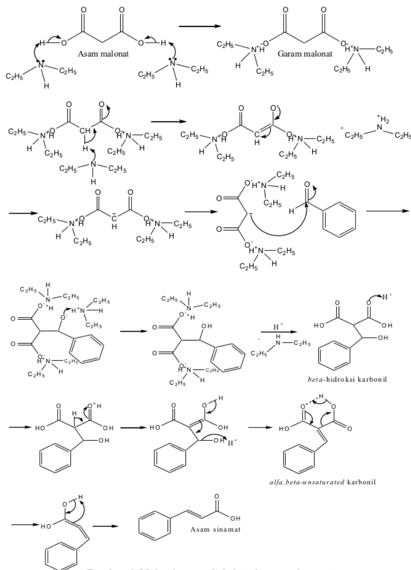
Gambar 6. Mekanisme reaksi sintesis asam sinamat.
