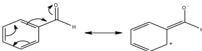
Gambar 2. Mekanisme resonansi yang terjadi pada benzaldehida
