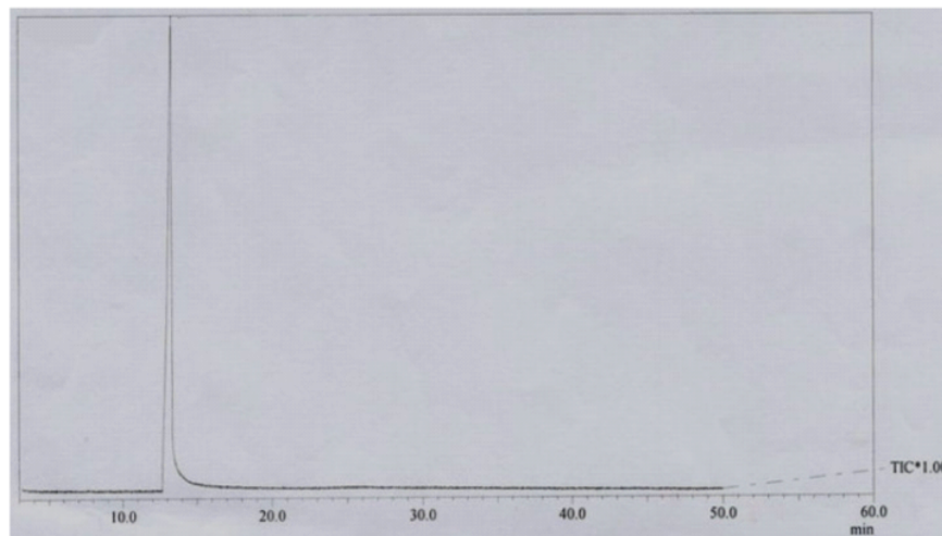
Gambar 4. Kromatogram kromatografi gas senyawa hasil sintesis.
