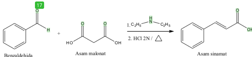
Gambar 1. Reaksi umum sintesis asam sinamat
