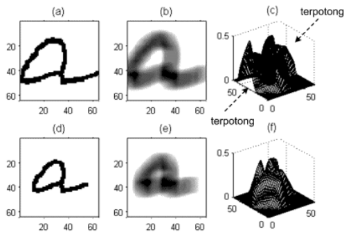
Gambar 7. Contoh pengaruh penekalaan huruf dalam template 64x64 piksel. (a) dan (d) penekalaan huruf ke 64x64 dan 48x48 piksel; (b) dan (e) masing-masing adalah hasil penapisan (a) dan (d), dengan tapis Gaussian 14x14 yang deviasi standarnya 10; (c) dan (f) masing-masing adalah gambaran jaring ( mesh ) (b) dan (e).
