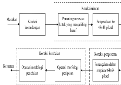
Gambar 6. Langkah-langkah pengolahan awal huruf.
