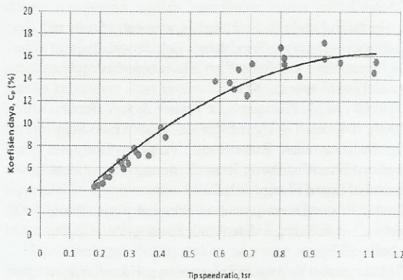
Gambar 6. Grafik hubungan C_p dan tsr diameter sudu 208 mm
