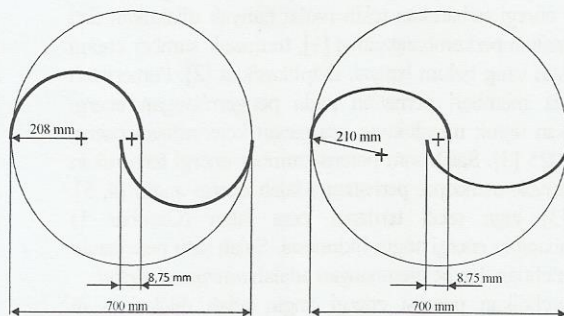
Gambar 4. Konfigurasi sudu kincir angin
