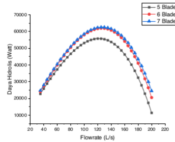
Gambar 8. Grafik Flowrate-Daya Hidrolis pada Variasi Jumlah Blade
