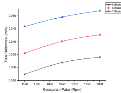
Gambar 14. Pengaruh Kecepatan Putar Impeler Terhadap Total Deformasi
