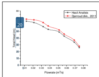
Gambar 4. Perbandingan Hasil Simulasi
