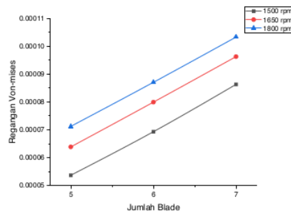
Gambar 14. Pengaruh Jumlah Blade Impeler terhadap Regangan Maksimum
