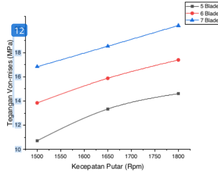
Gambar 12. Pengaruh Kecepatan Putar Impeler Terhadap Tegangan Maksimum
