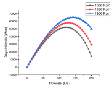
Gambar 8. Grafik Flowrate-Daya Hidrolis pada Variasi Kecepatan Putar
