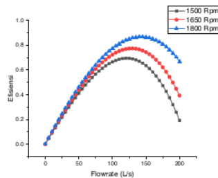
Gambar 9. Grafik Flowrate-Efisiensi pada Variasi Kecepatan Putar
