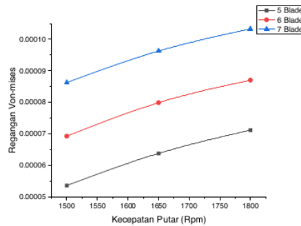
Gambar 13. Pengaruh Kecepatan Putar Impeler Terhadap Regangan Maksimum
