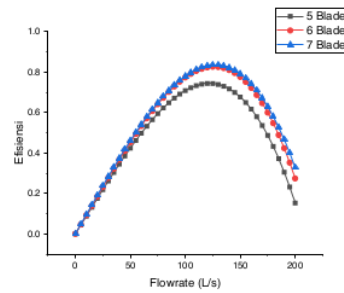
Gambar 10. Grafik Flowrate-Efisiensi pada Variasi Kecepatan Putar
