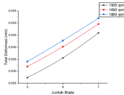
Gambar 15. Pengaruh Jumlah Blade Impeler terhadap Total Deformasi Maksimum
