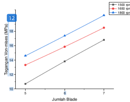
Gambar 13. Pengaruh Jumlah Blade Impeler terhadap Tegangan Maksimum
