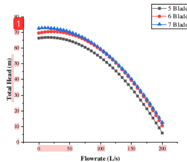
Gambar 7. Grafik Flowrate-Total Head pada Variasi Jumlah Blade
