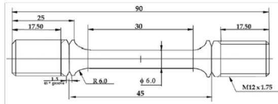
Gambar 2: Spesimen uji tarik paduan 800H [3].
