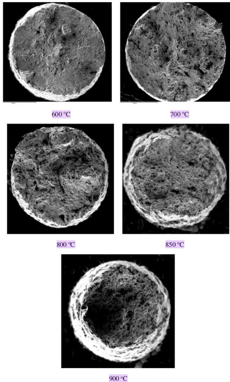
Gambar 6: Profil patahan spesimen melalui pengamatan SEM.
