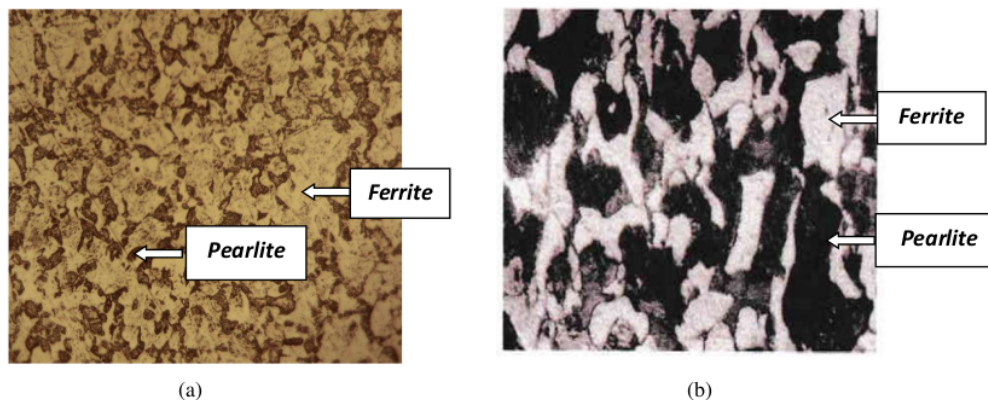
Gambar 4. (a). Struktur mikro baja AISI 1045 sebelum dilakukan proses heat treatment dengan pembesaran 222x, (b) Foto struktur mikro baja AISI 1045 sebelum dilakukan proses heat treatment dengan pembesaran 800x, Nital 2% [13].
