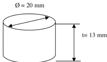
Gambar 1. Dimensi spesimen uji kekerasan Vickers
