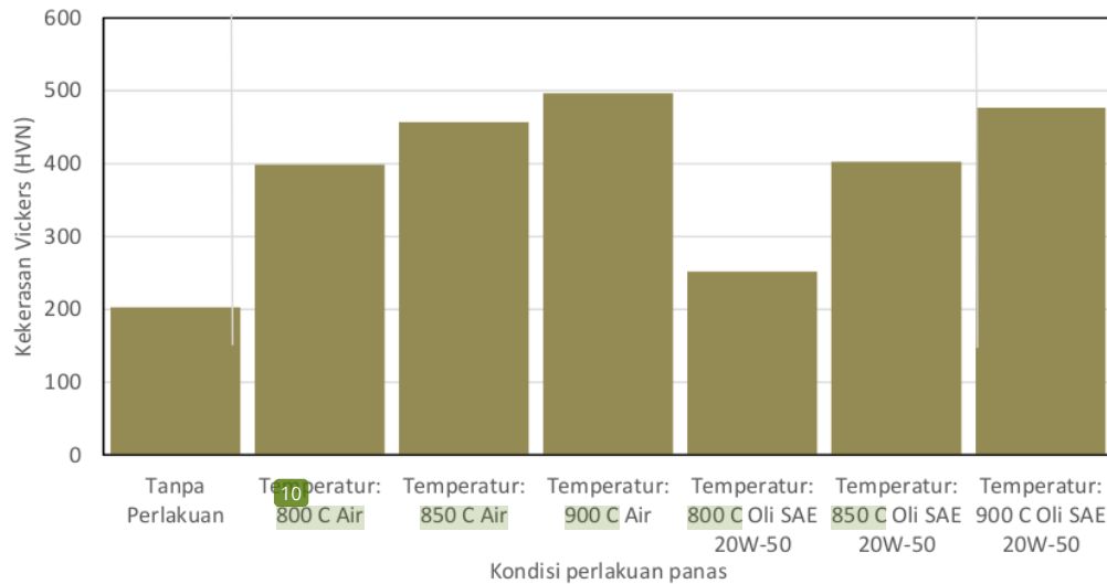
Gambar 3. Grafik perbandingan tingkat kekerasan baja AISI 1045 pada variasi temperatur quenching dan media pendingin
