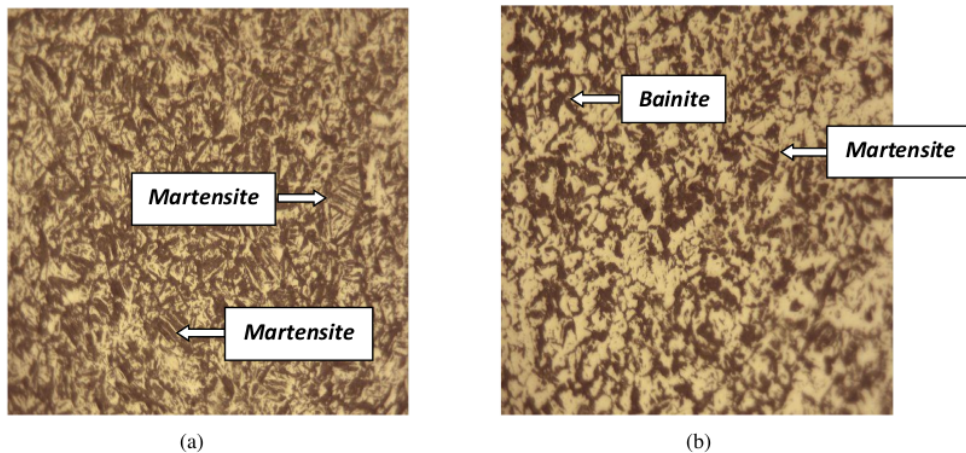
Gambar 6. (a) Struktur mikro baja AISI 1045 setelah dilakukan proses quenching pada suhu 900°C dengan holding time selama 25 menit menggunakan media pendingin air, pembesaran 222x, (b) Struktur mikro baja AISI 1045 setelah dilakukan proses quenching pada suhu 800°C dengan holding time selama 25 menit menggunakan media pendingin oli SAE 20W-50, pembesaran 222x.
