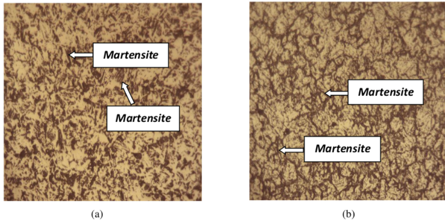
Gambar 5. (a) Struktur mikro baja AISI 1045 setelah dilakukan proses quenching pada suhu 800°C dengan holding time selama 25 menit menggunakan media pendingin air, pembesaran 222x, (b) Struktur mikro baja AISI 1045 setelah dilakukan proses quenching pada suhu 850°C dengan holding time selama 25 menit menggunakan media pendingin air, pembesaran 222x.
