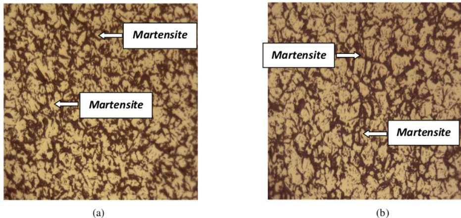
Gambar 7. (a) Struktur mikro baja AISI 1045 setelah dilakukan proses quenching pada suhu 850°C dengan holding time selama 25 menit menggunakan media pendingin oli SAE 20W-50, pembesaran 222x, (b) Struktur mikro baja AISI 1045 setelah dilakukan proses quenching pada suhu 900°C dengan holding time selama 25 menit menggunakan media pendingin oli SAE 20W-50, pembesaran 222x.
