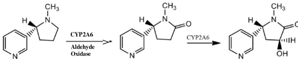
Gambar 1. Jalur utama metabolisme nikotin oleh enzim CYP2A6 (1).
