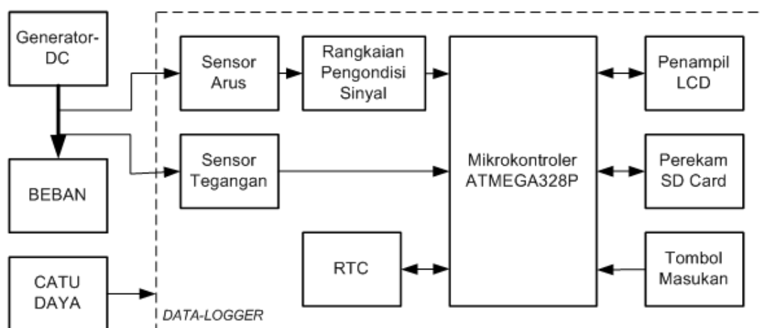
Gambar 1. Diagram Kotak Sistem.
