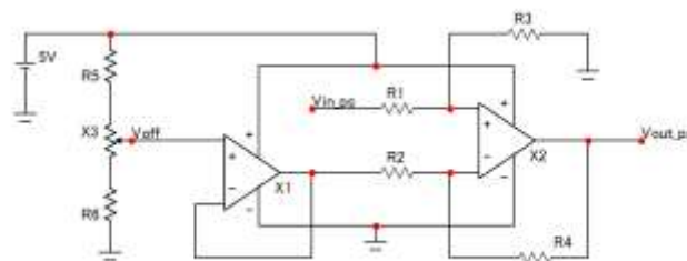
Gambar 5. Rangkaian Pengondisi Sinyal Besaran Arus.
