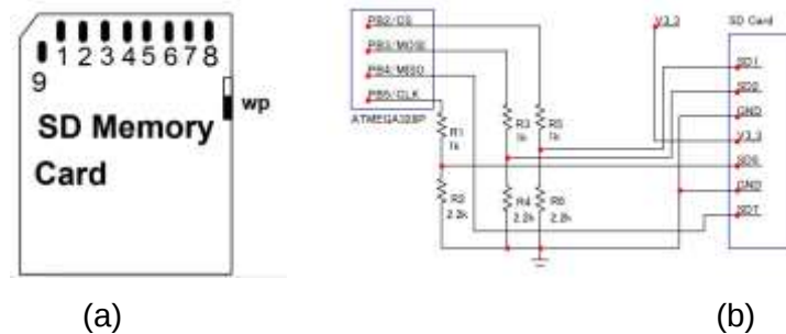
Gambar 10.(a) Standar Penomoran Terminal SD Card (SD Group, 2013). (b). Hubungan SD Card dengan mikrokontroler.
