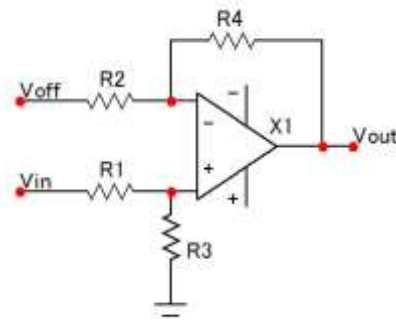
Gambar 4. Rangkaian penguat selisih tegangan (Boylestad, 2011)
