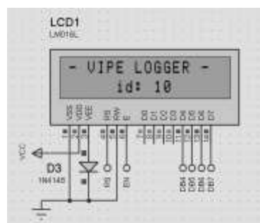
Gambar 9. Rangkaian Penampil LCD.
