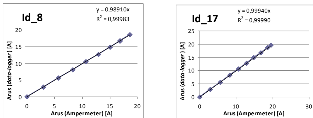
Gambar 13 Kurva perbandingan antara arus hasil pengukuran dengan amperemeter dan arus hasil pengukuran data-logger, untuk dua data logger .
