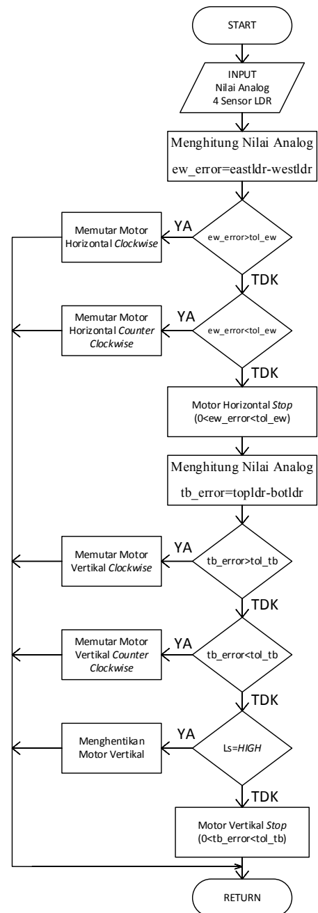
Gambar 6. Diagram alir sistem pelacak matahari
