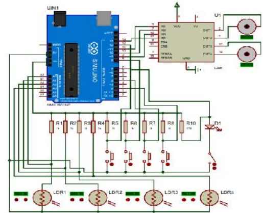
Gambar 5. Rancangan elektronis sistem pelacak matahari
