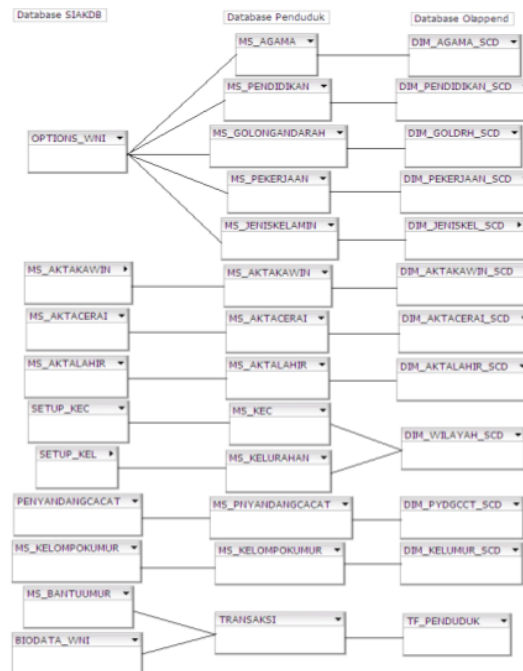
Gambar 1. Alur proses pembentukan tabel dan proses transformasi data
