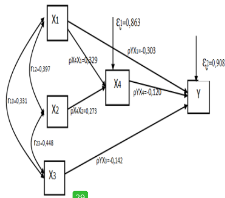
29 Gambar 5. Hubungan Kausal Empiris Variabel X1, X2, X3, dan X4 terhadap Y
