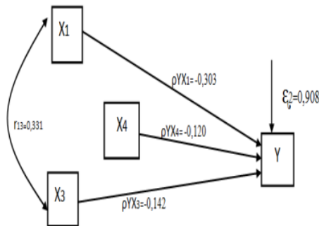
18 Gambar 4. Hubungan Kausal Empiris Substruktur 2 Variabel X1, X3, dan X4 terhadap Y
