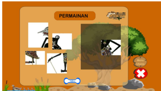
Gambar 5. Halaman Permainan
