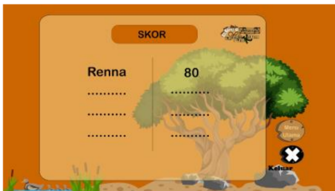
Gambar 10. Halaman Skor
