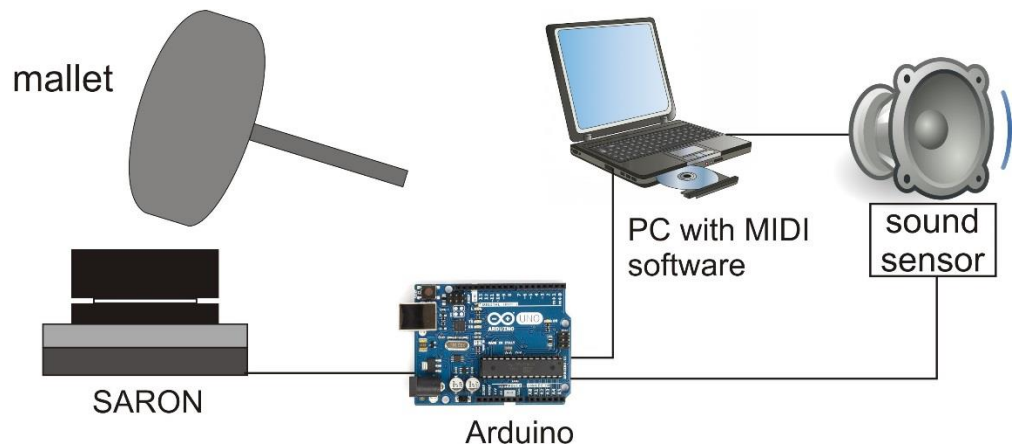
Gambar 2. Skema piranti pendukung Gamelan Listrik
