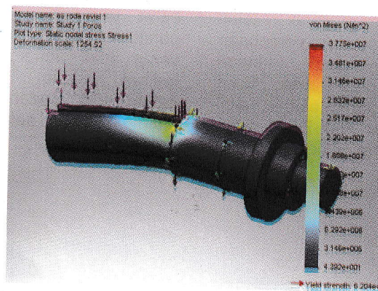
Gambar 12. Hasil Analisa Kekuatan Poros Roda
