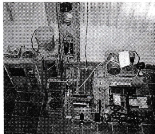
Gambar 12. Plant proses produksi
