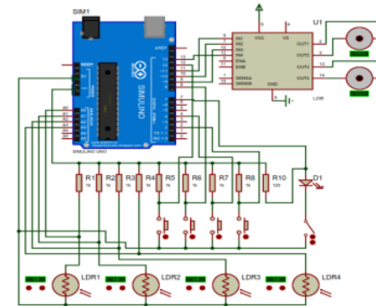
Gambar 5. Rancangan elektronis sistem pelacak matahari
