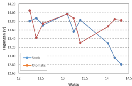
Gambar 10. Hasil pengujian tegangan
