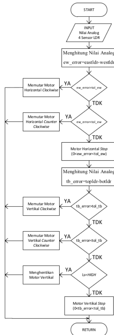
Gambar 6. Diagram alir sistem pelacak matahari
