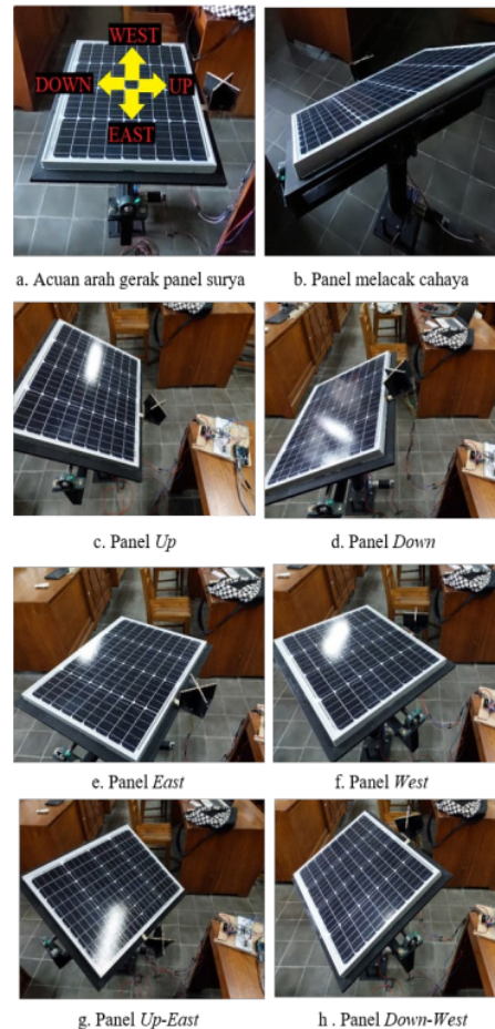
Gambar 8. Pengujian gerakan motor mengikuti arah cahaya
