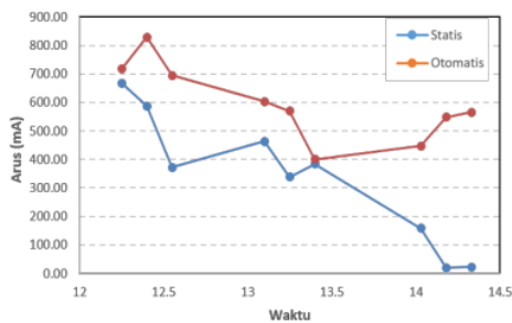
Gambar 9. Hasil pengujian arus
