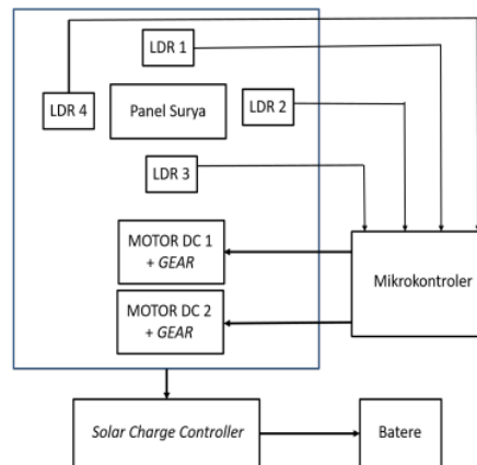
Gambar 1. Blok diagram sistem pelacak sinar matahari
