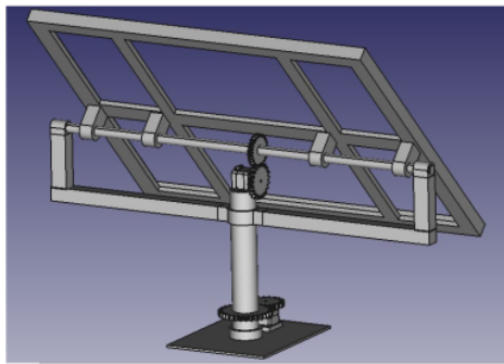
Gambar 4. Rancangan rangka pelacak matahari
