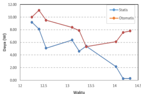
Gambar 11. Hasil pengujian daya
