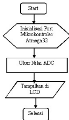
Gambar 2. Flowchart pengukuran kekeruhan air sungai
