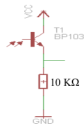
Gambar 3. Rangkaian fototransistor.
