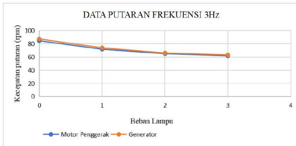
Gambar 18. Data putaran dengan frekuensi 3Hz
