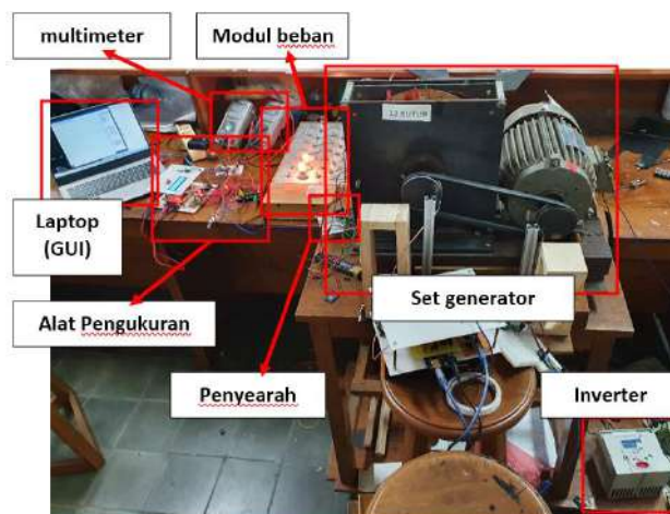
Gambar 6. Keseluruhan sistem pengukuran daya keluaran
