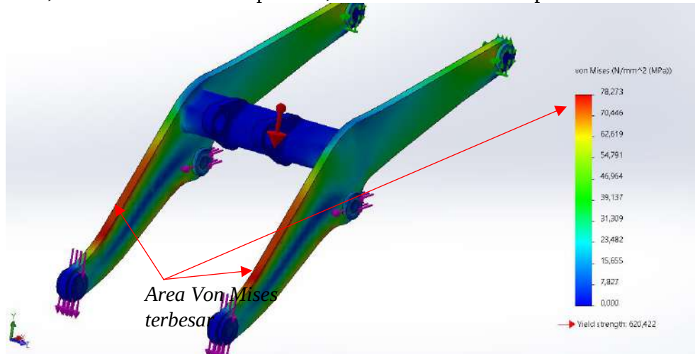
Gambar 5. Distribusi tegangan Von Mises posisi 1
