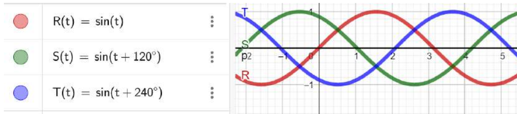
Gambar 15. Protokol Konstruksi untuk visualisasi sumber tegangan 3 fase
