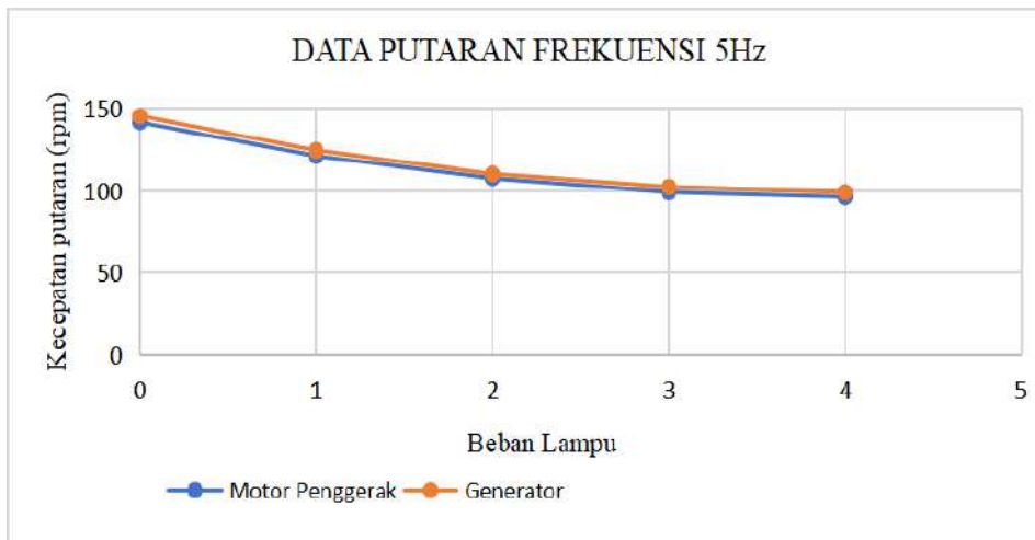
Gambar 20. Data putaran dengan frekuensi 5Hz
