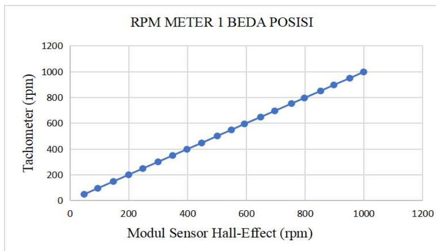
Gambar 16. Pengukuran rpm meter 1 beda posisi
