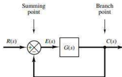
Gambar 1. Blok Diagram Sistem Loop Tertutup
