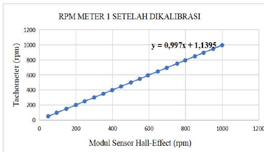
Gambar 13. Persamaan rpm meter 1 setelah dikalibrasi
