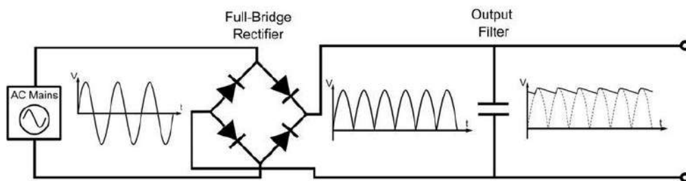
Gambar 2. Skema Penyearah Jembatan Penuh ( Full-Bridge Rectifier )
