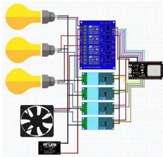
Gambar 3 Rangkain wiring NodeMCU
