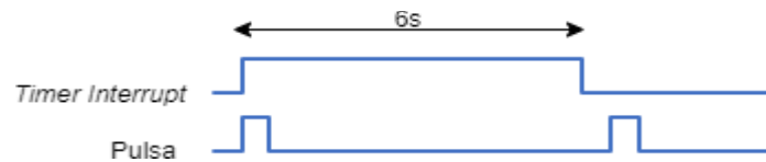
Gambar 7. Keadaan rpm nol
