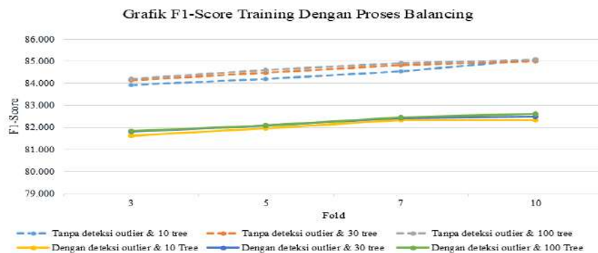
Gambar 15. Grafik hasil f1-score training dengan proses balancing
