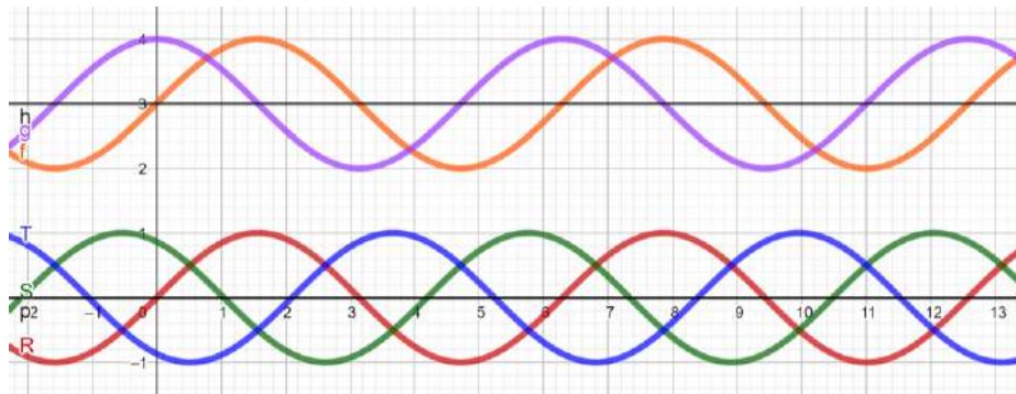
Gambar 11. Visualisasi sumber tegangan 2 fase dan sumber tegangan 3 fase Sumber tegangan dalam bentuk vektor
