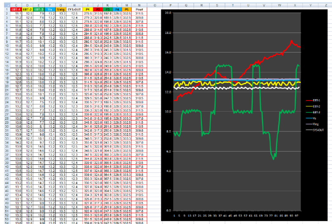
Gambar 11. Perolehan Data beserta Grafik Simulasi Fluktuasi multisumber EBT, Power Storage , dan Keluaran Sumber ( V_s ) dan Beban ( V_b )
