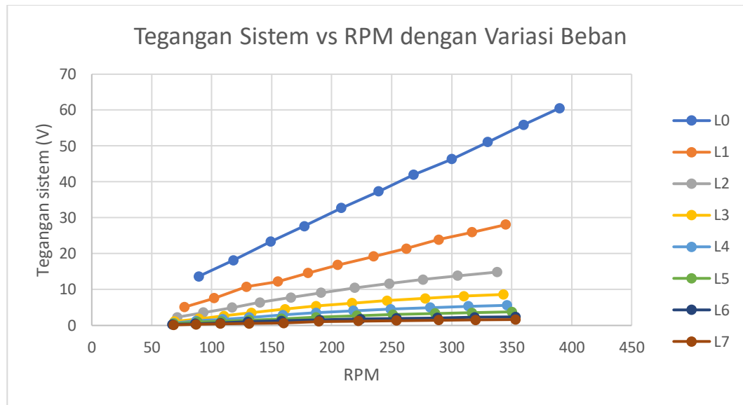
Gambar 13. Grafik tegangan sistem vs RPM dengan variasi beban
