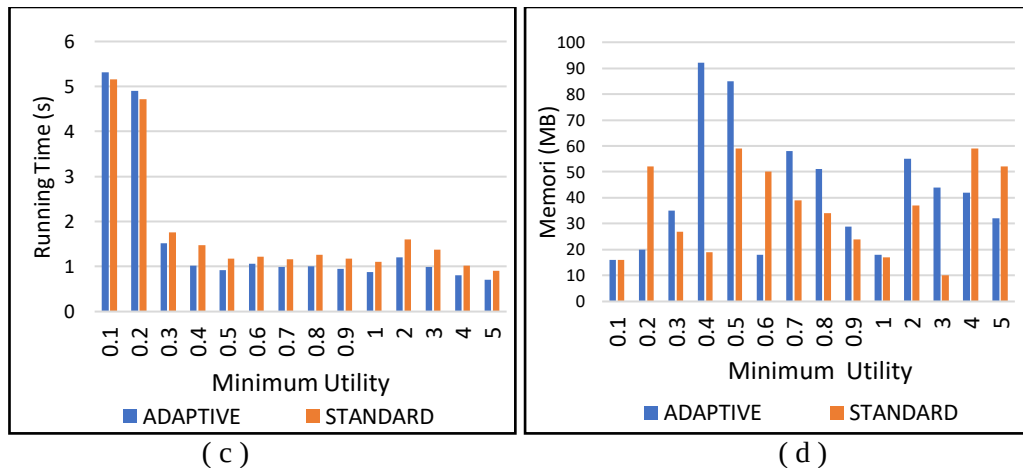
Gambar 2. Perbandingan jumlah itemset , total utility (baris pertama), running time dan penggunaan memori (baris kedua) dari metode BPSO-standard dan BPSO-adaptive terhadap berbagai nilai minimum utility
