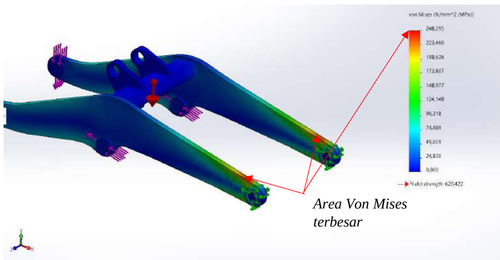
Gambar 5. Distribusi tegangan Von Mises posisi 1
