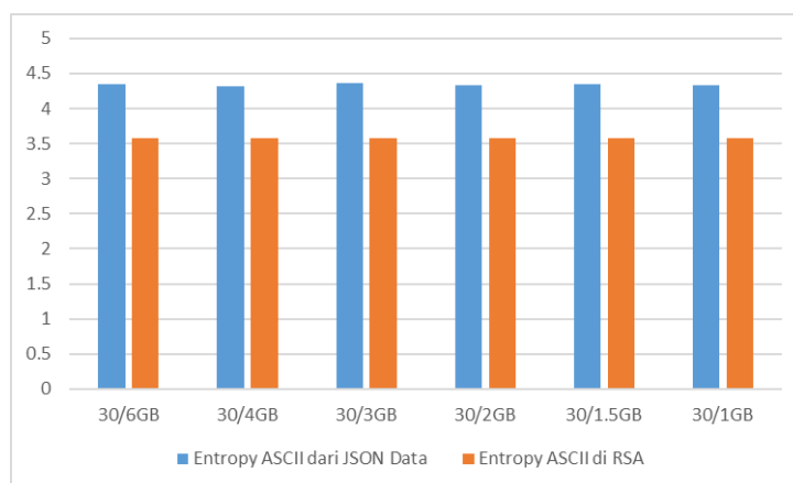
Gambar 7. Entropy untuk Enkripsi AES dan RSA pada berbagai Ukuran Memori Smartphone.
