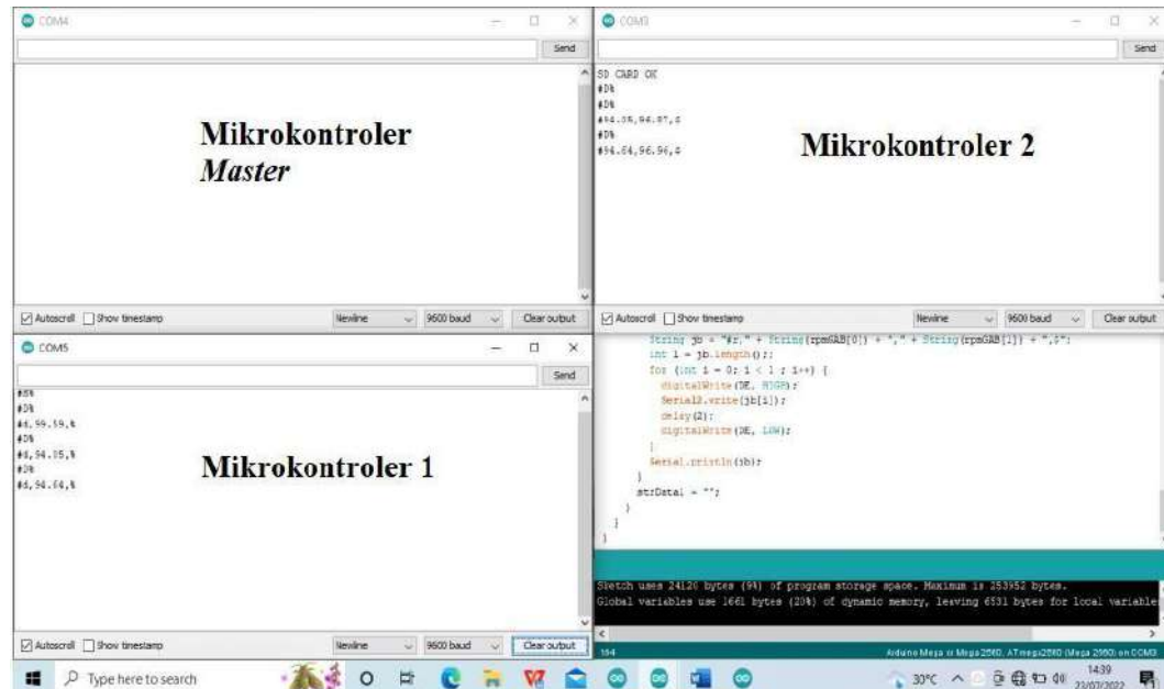
Gambar 31. Komunikasi data mikrokontroler 1 dan mikrokontroler 2
