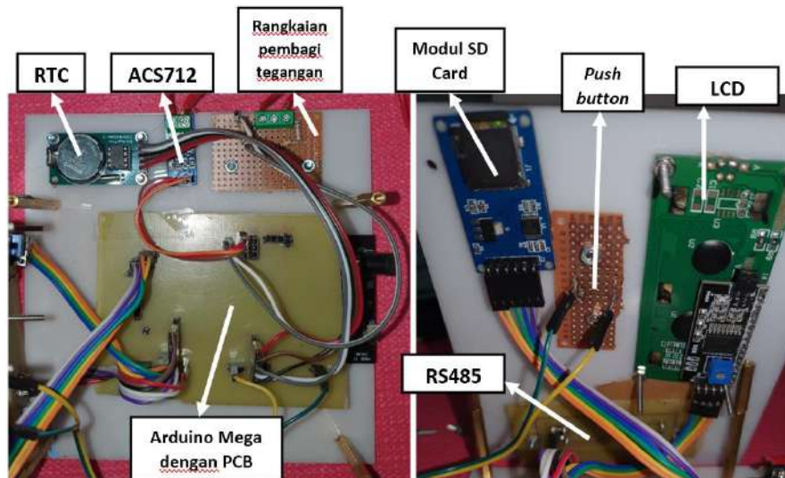
Gambar 8. Bagian dalam kotak
