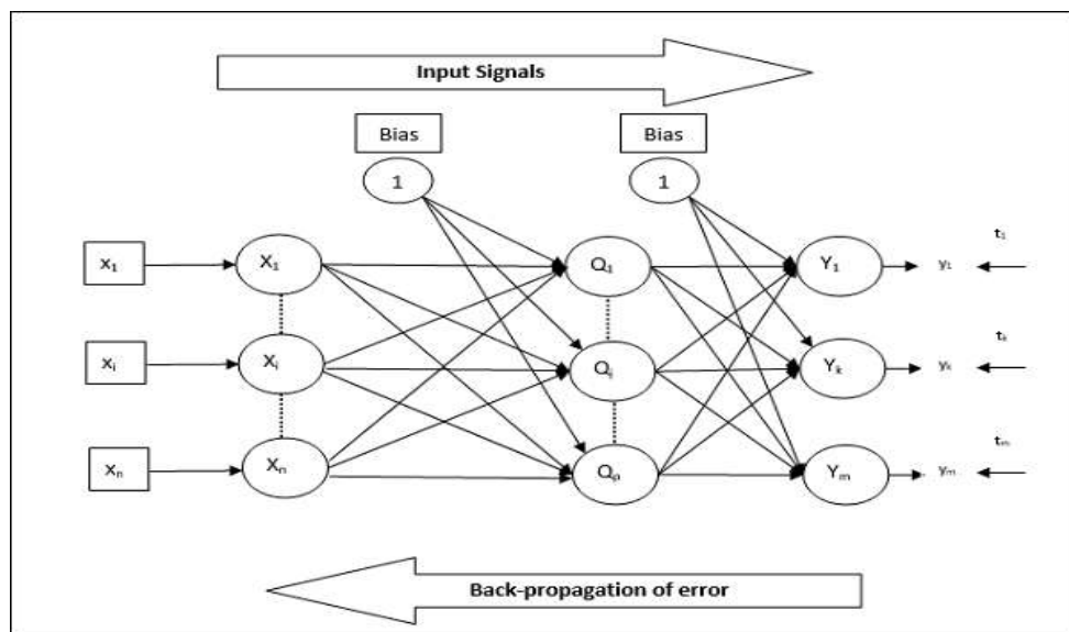
Gambar 2. Contoh arsitektur Jaringan Syaraf Tiruan Perambatan Balik
