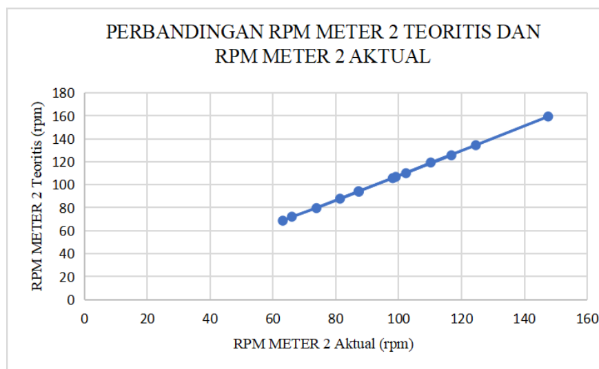
Gambar 21. Perbandingan rpm meter 2 teoritis dan rpm meter 2 aktual
