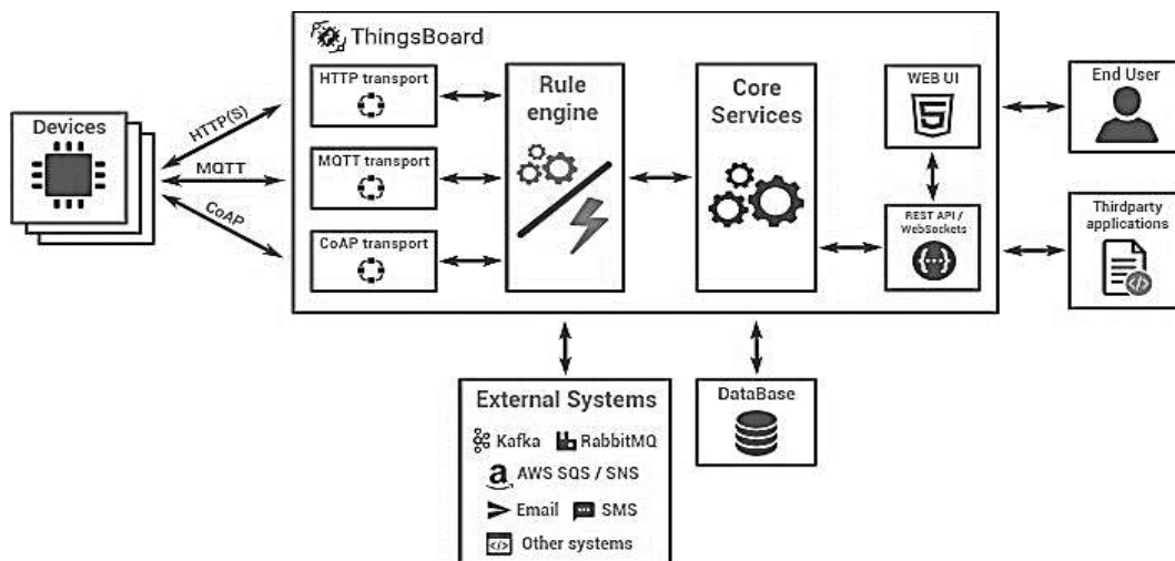
Gambar 1. Arsitektur ThingsBoard (Saptaji, 2019).
