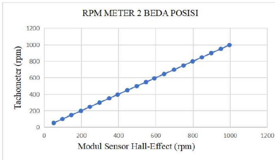
Gambar 17. Pengukuran rpm meter 2 beda posisi
