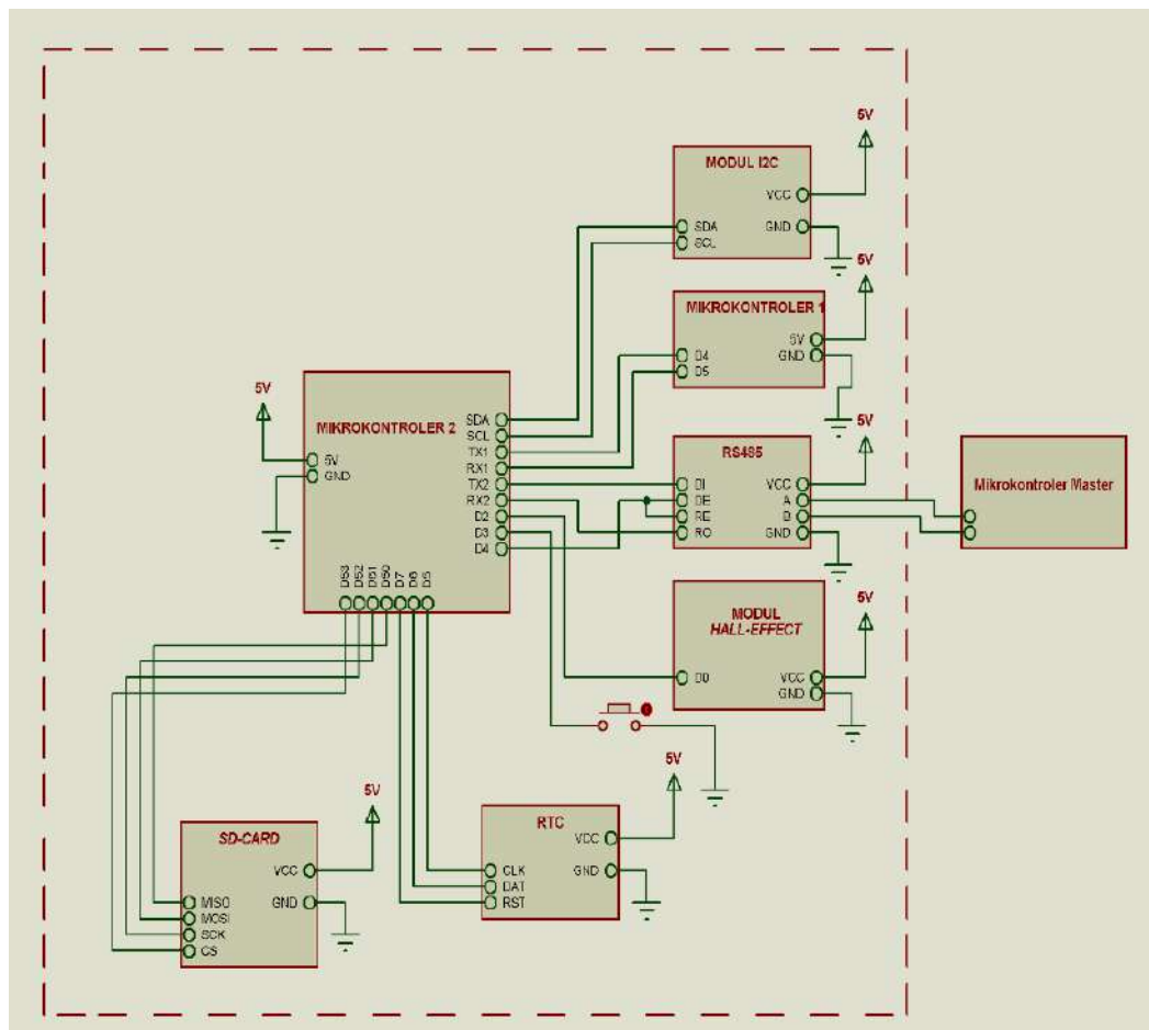
Gambar 3. Rangkaian mikrokontroler 2
