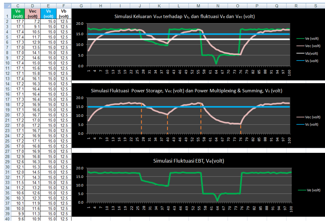
Gambar 9. Perolehan Data beserta Grafik Simulasi Fluktuasi per unit sumber EBT, Power Storage , dan Keluaran Sumber ( V_s ) dan Beban ( V_b )
