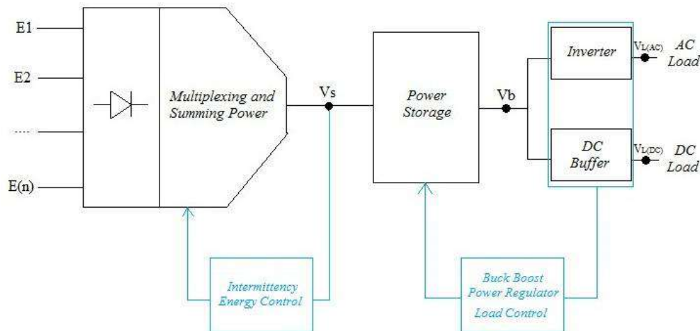
Gambar 3. Blok Diagram Sistem Antarmuka Multisumber EBT
