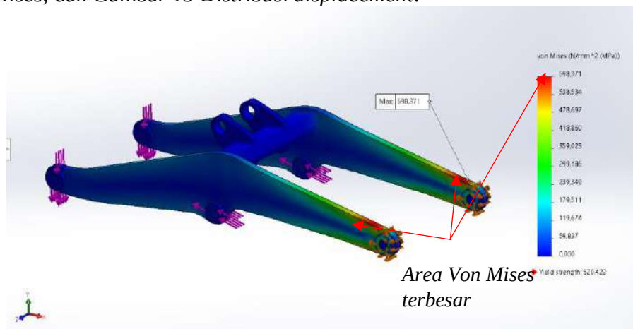
Gambar 12. Distribusi tegangan Von Mises setelah pertambahan panjang
