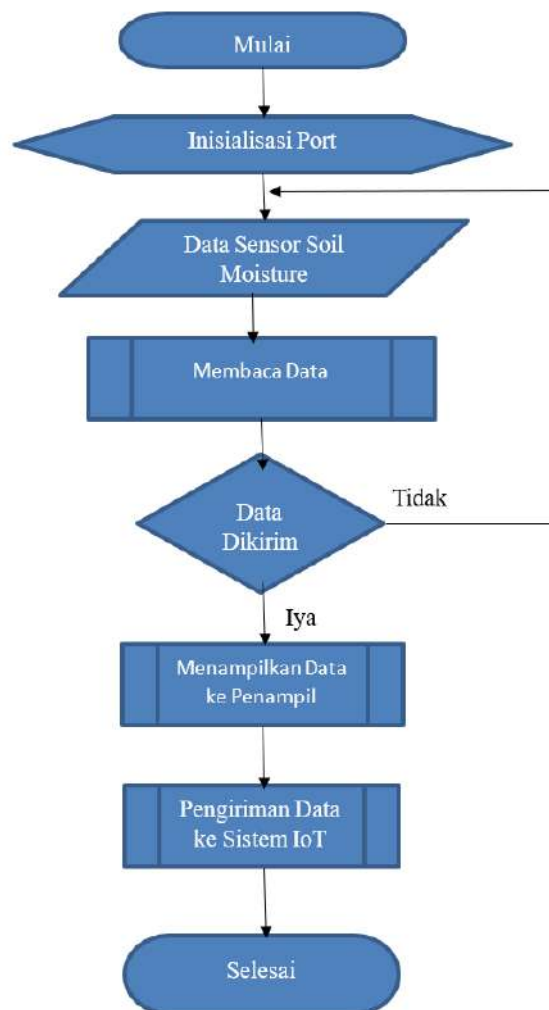
Gambar 2. Diagram alir utama pemrosesan data
