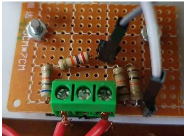
Gambar 34. Implementasi rangkaian pembagi tegangan
