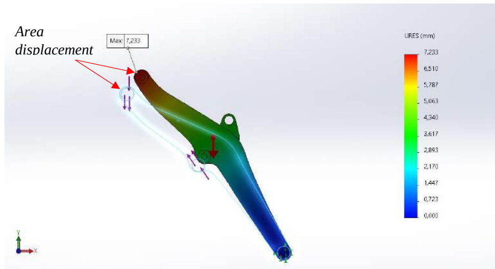
Gambar 11. Distribusi displacement posisi 3
