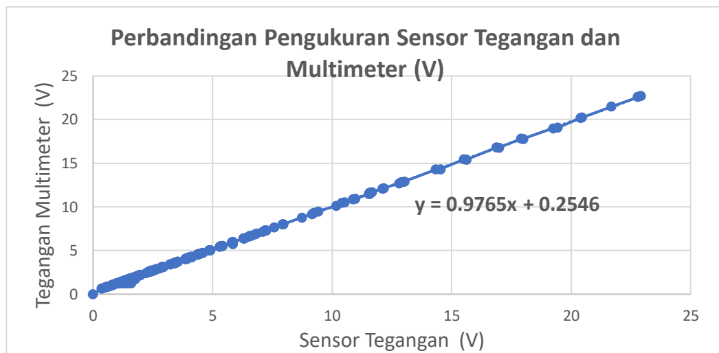
Gambar 35. Grafik kalibrasi sensor tegangan
