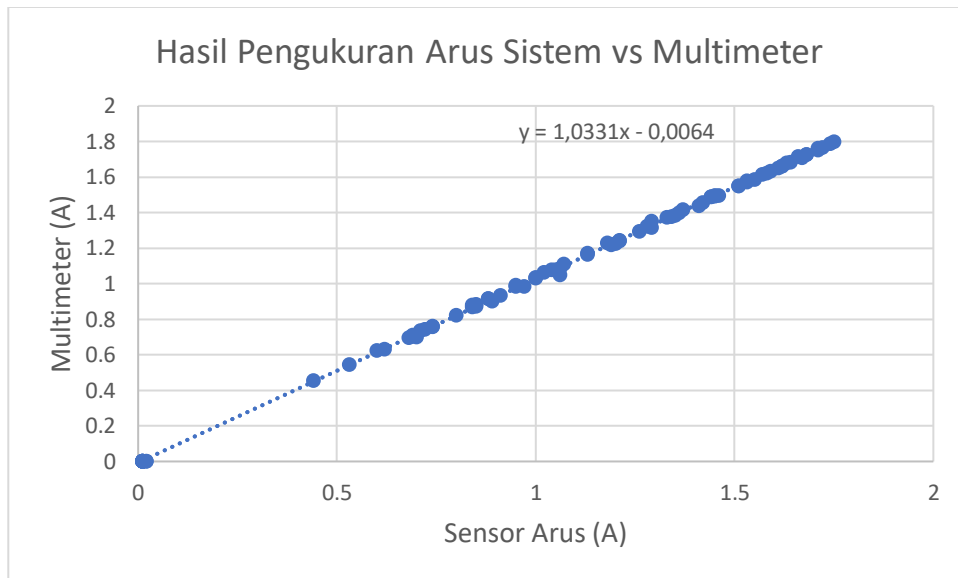
Gambar 17. Grafik perbandingan hasil pengukuran arus
