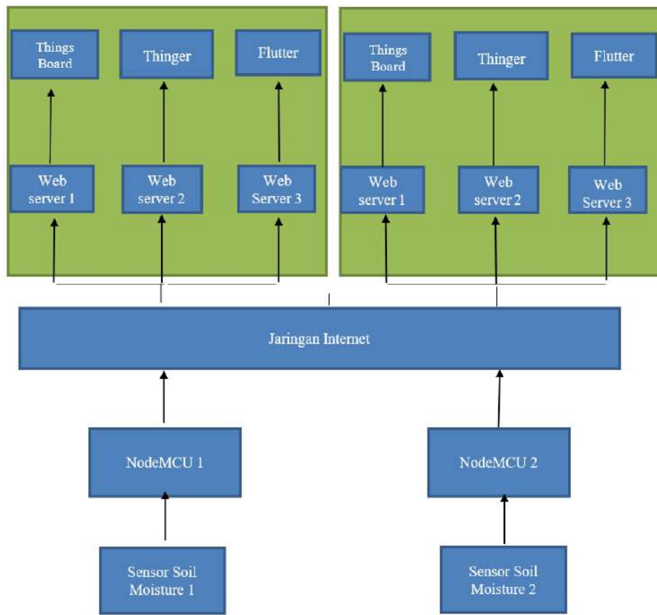
Gambar 1. Diagram blok ketiga sistem transmisi data dengan sensor dan NodeMCU
