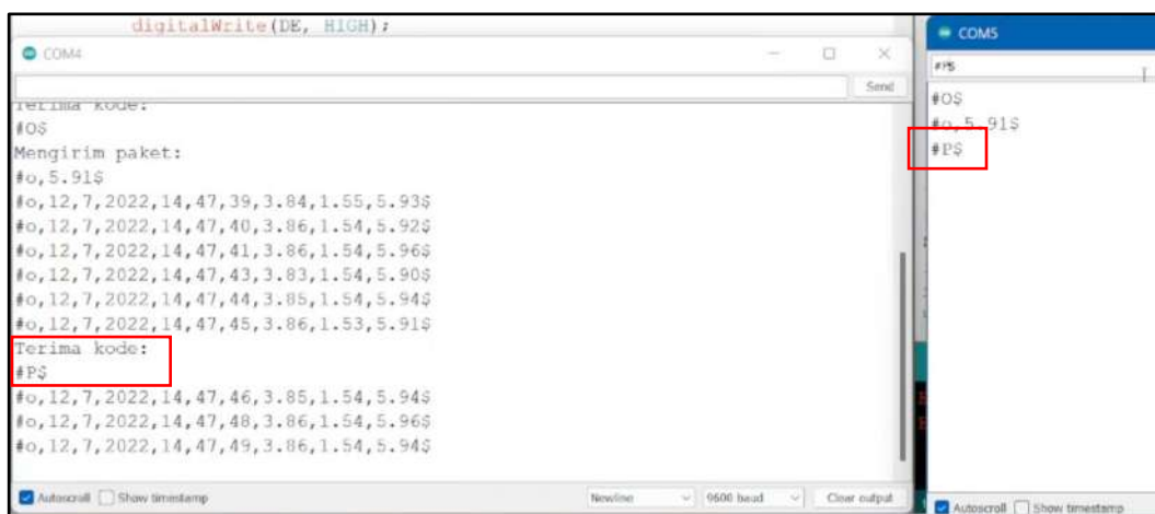
Gambar 27. Pengujian komunikasi RS485 slave dan master
