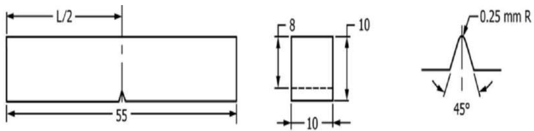
Gambar 5. Rancangan spesimen pengujian impact
