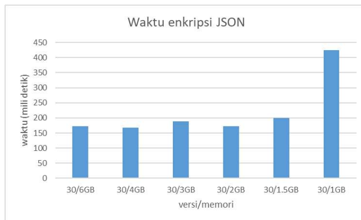
Gambar 5. Waktu Enkripsi Proses Enkripsi dengan AES untuk berbagai Ukuran Memori Smartphone.
