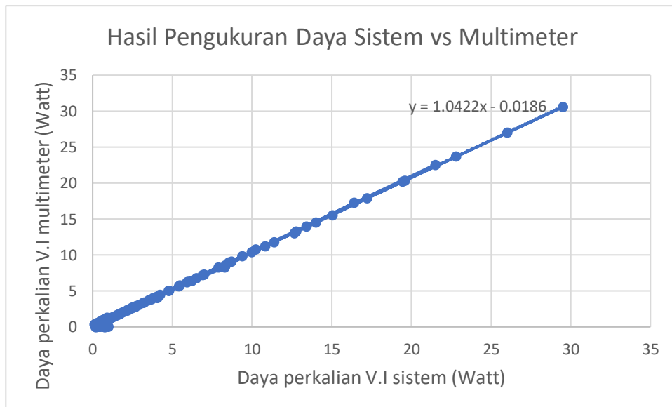
Gambar 18. Grafik perbandingan hasil pengukuran daya
