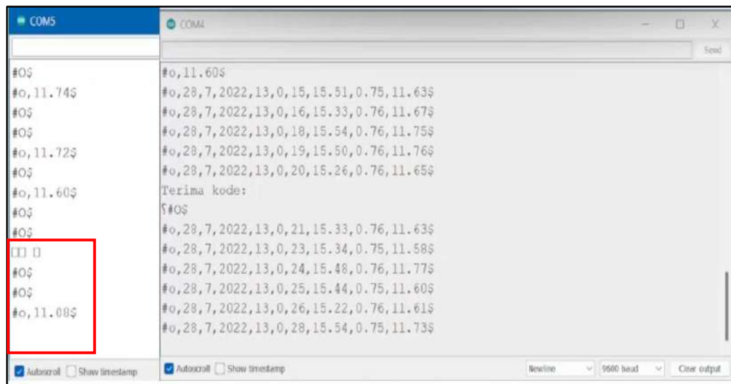
Gambar 30. Pengujian komunikasi RS485 slave dan master
