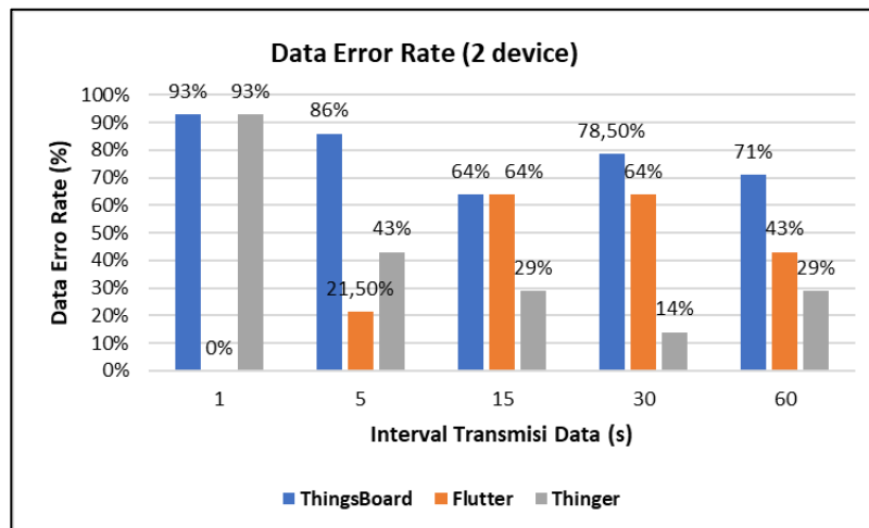
Gambar 6. Data error rate untuk pengukuran transmisi data dari 2 device .
