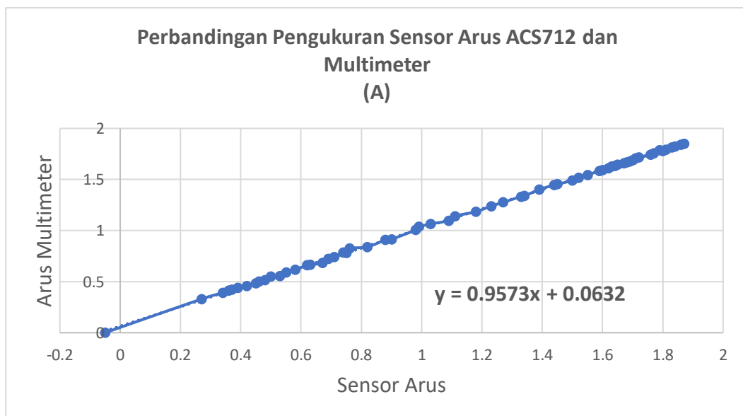
Gambar 32. Grafik kalibrasi sensor arus
