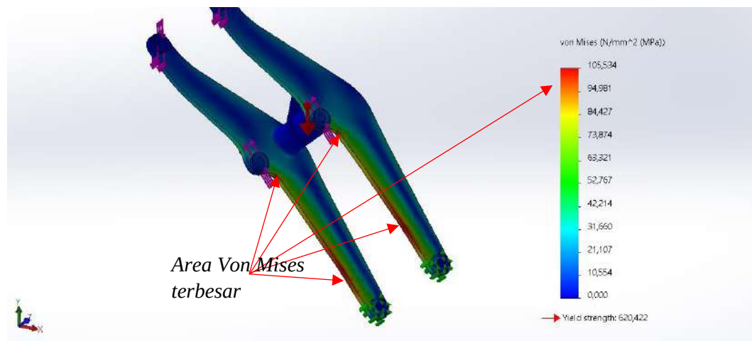
Gambar 7. Distribusi tegangan Von Mises posisi 3
