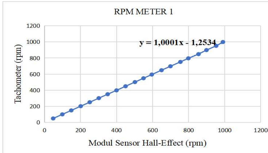
Gambar 12. Persamaan rpm meter 1 sebelum kalibrasi
