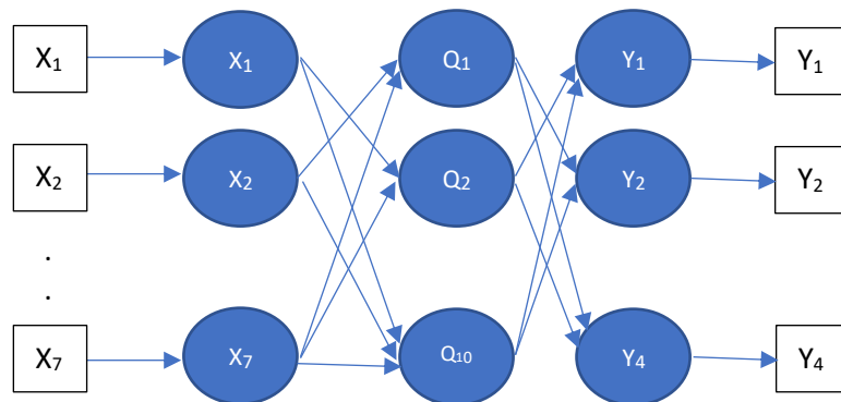
Gambar 3. Arsitektur Jaringan syaraf tiruan untuk pengawasandi blok linear (7,4)
