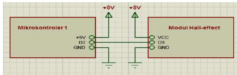
Gambar 2. Rangkaian mikrokontroler 1
