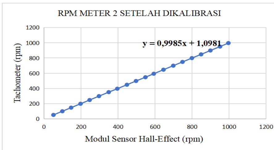
Gambar 15. Persamaan rpm meter 2 setelah dikalibrasi
