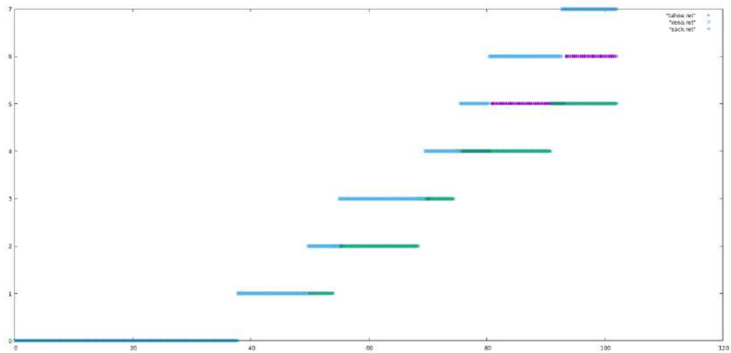
Gambar 7. Grafik retransmit TCP Tahoe, Reno, New Reno, SACK tanpa trafik pengganggu
