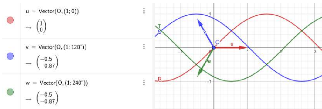
Gambar 19. Sumber tegangan AC 3 fase dalam bentuk vektor dengan sudut antar fase 120 derajat
