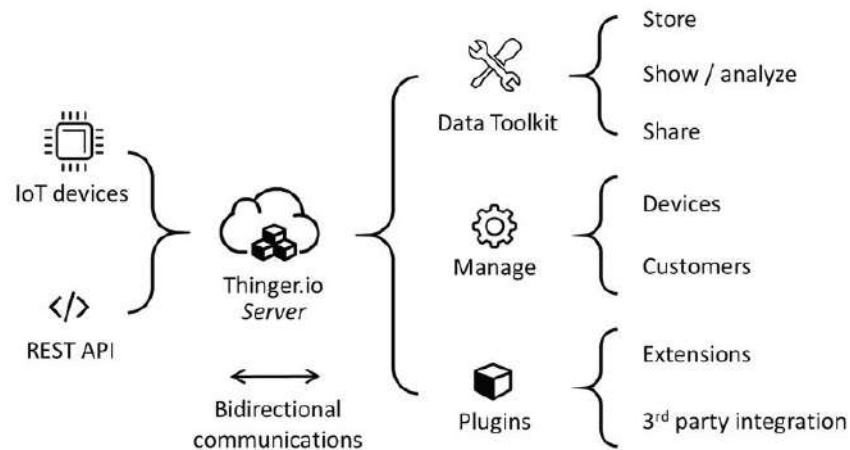
Gambar 2. Fitur utama platform IoT Thingier.io (Thingier.io, 2021)
