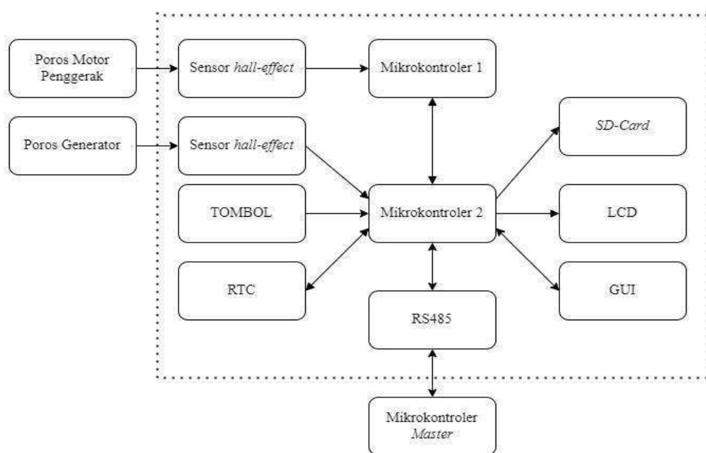
Gambar 1. Diagram blok sistem
