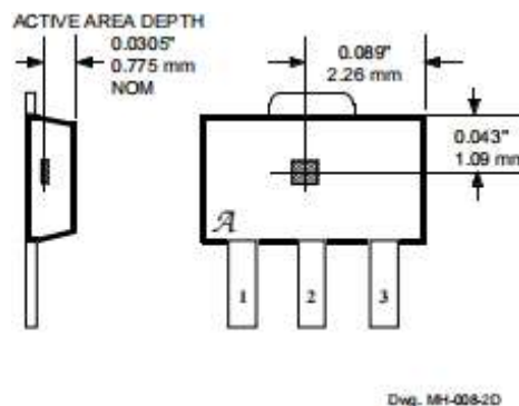
Gambar 1. Area aktif sensor
