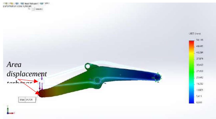
Gambar 13. Distribusi Displacement setelah pertambahan Panjang
