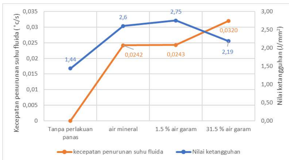
Gambar 104. Hubungan kecepatan penurunan suhu fluida terhadap nilai ketangguhan Baja AISI 1045
