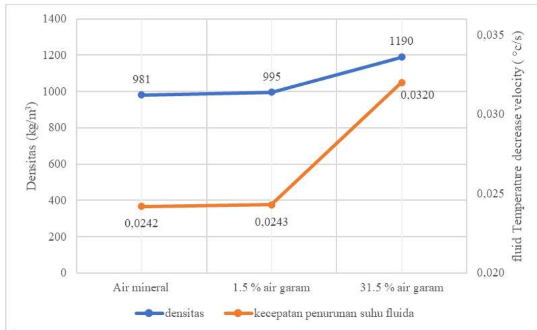
Gambar 8. Hubungan densitas dan penurunan suhu pada fluida
