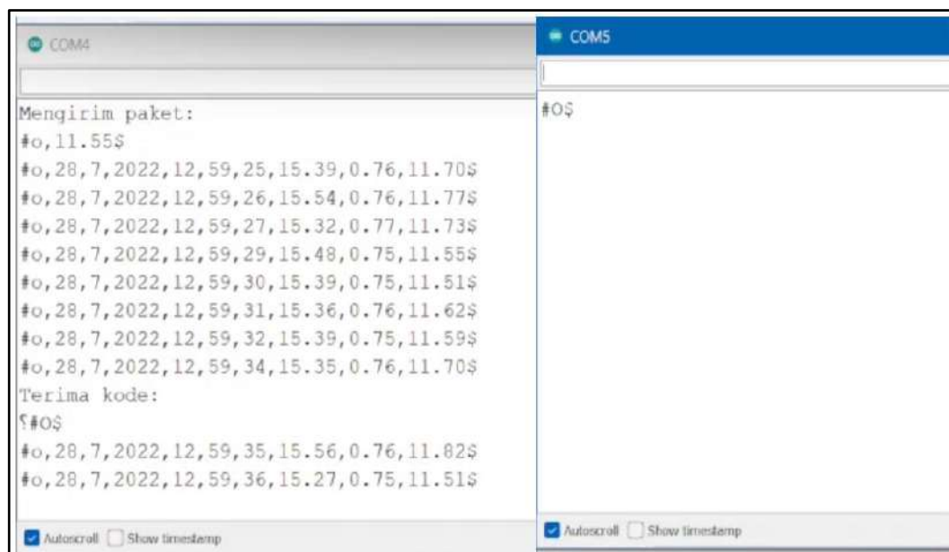
Gambar 29. Pengujian komunikasi RS485 slave dan master
