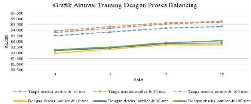
Gambar 14. Grafik hasil akurasi training dengan proses balancing
