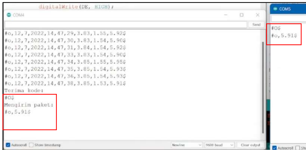
Gambar 26. Pengujian komunikasi RS485 slave dan master
