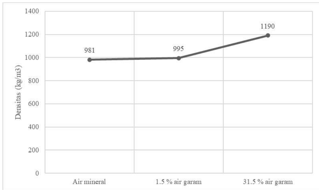
Gambar 6. Hubungan densitas dan media quenching
