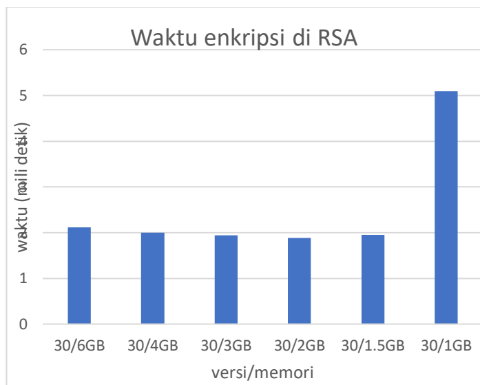
Gambar 6. Waktu Enkripsi Proses Enkripsi Data dengan RSA untuk berbagai Ukuran Memori Smartphone.
