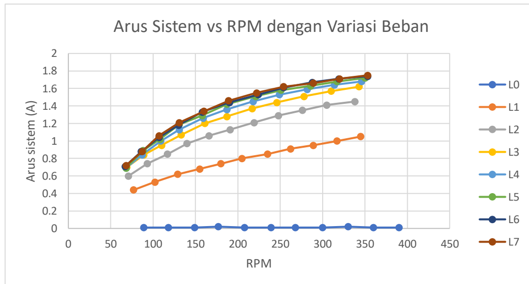
Gambar 14. Grafik arus sistem vs RPM dengan variasi beban
