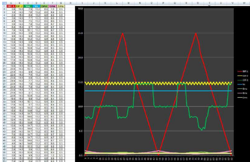
Gambar 10. Data beserta Grafik Simulasi Proses Buck Boost Regulator Pada Setiap EBT
