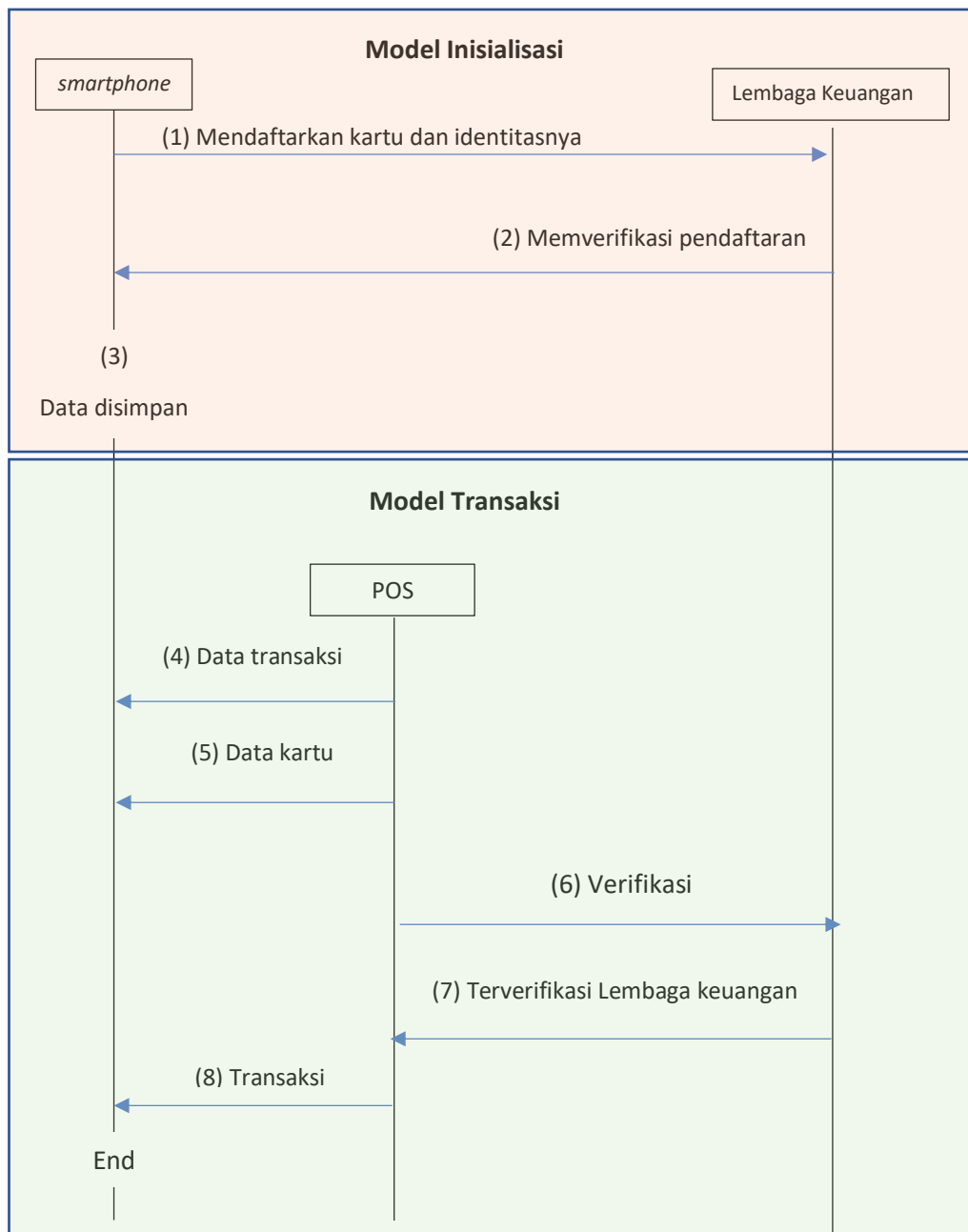
Gambar 2. Gambaran umum model inisialisasi dan transaksi.
