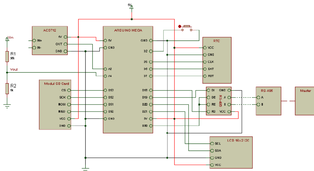
Gambar 3. Pengkabelan sistem pengukuran
