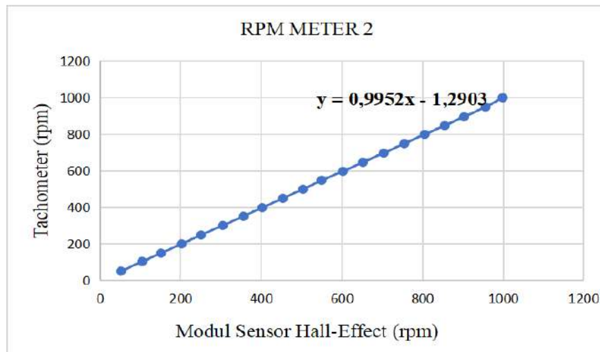
Gambar 14. Persamaan rpm meter 2 sebelum kalibrasi
