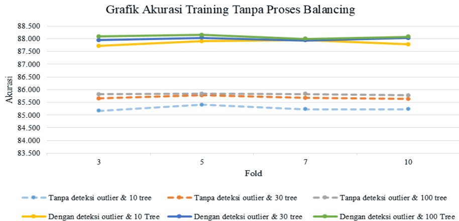
Gambar 12. Grafik hasil akurasi training tanpa proses balancing
