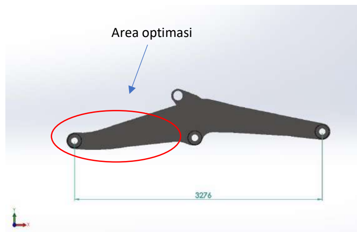
Gambar 4. Lift arm sesudah pertambahan panjang
