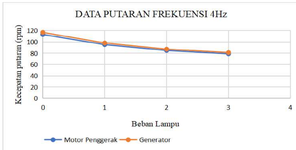
Gambar 19. Data putaran dengan frekuensi 4Hz
