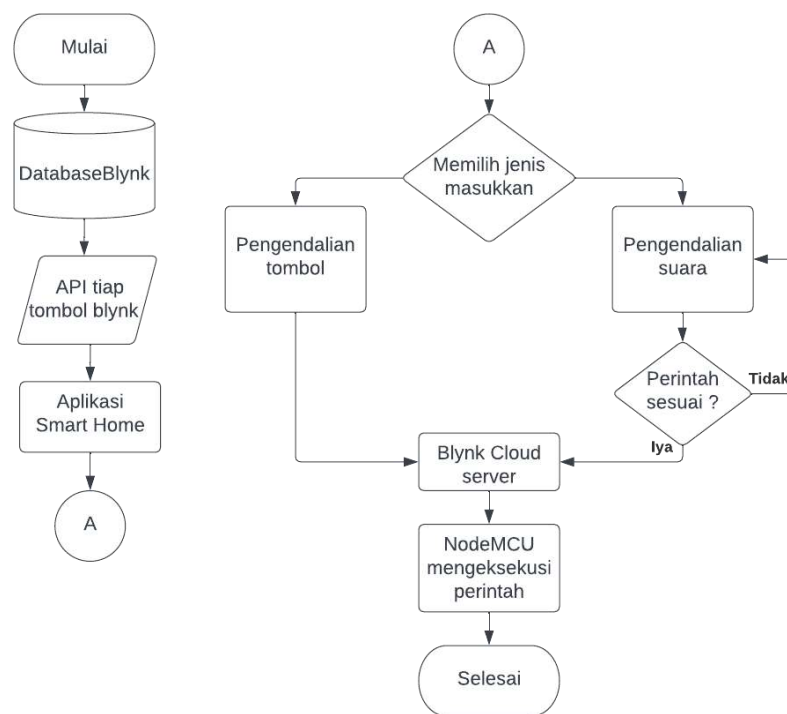
Gambar 4 Diagram alir sistem pengendalian
