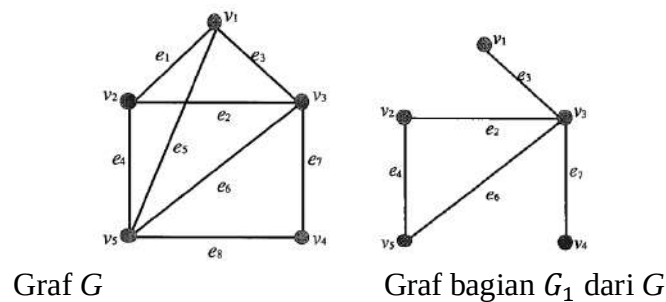
Gambar 3. Contoh graf bagian dari graf.
