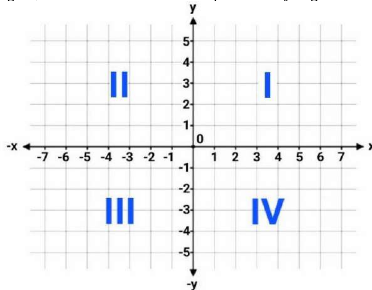
Gambar 3. Kuadran koordinat kartesius
