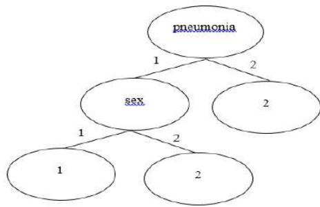
Gambar 3. Tree dengan node ke-5
