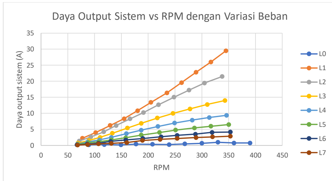
Gambar 15. Grafik daya keluaran sistem vs RPM dengan variasi beban
