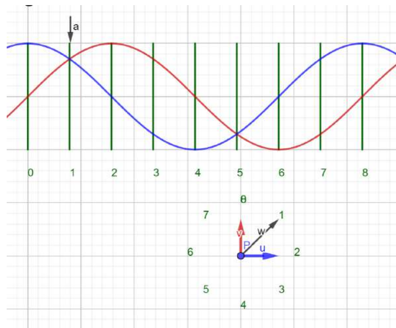
Gambar 18. Arah medan magnet pada motor 2 fase
