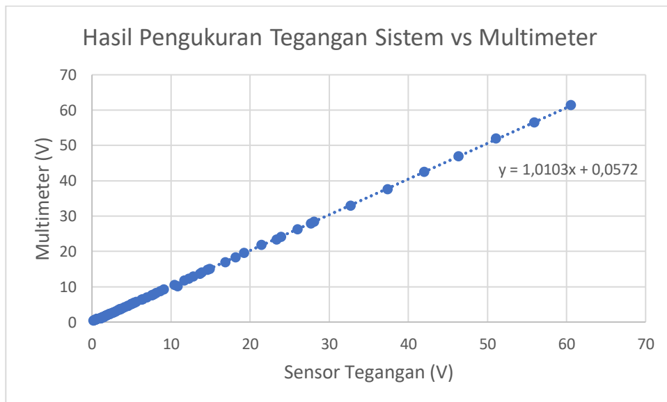
Gambar 16. Grafik perbandingan hasil pengukuran tegangan
