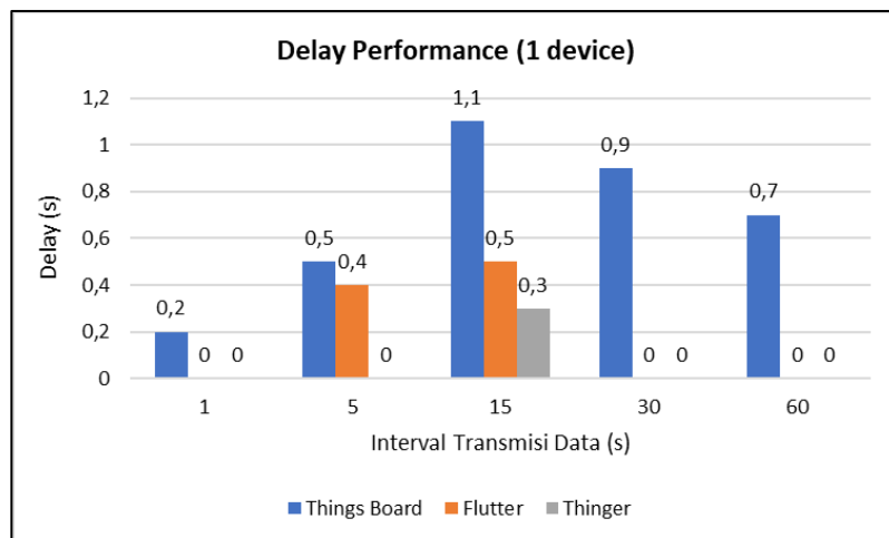
Gambar 3. Delay performance untuk pengukuran transmisi data dari 1 device .
