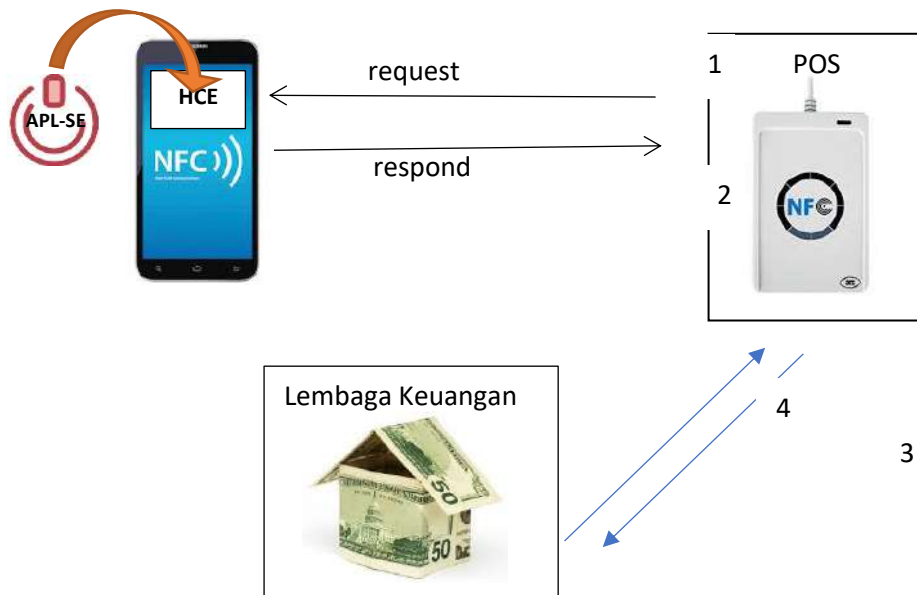
Gambar 1. Rancangan Arsitektur APL-SE (Lucia Nugraheni Harnaningrum et al., 2022)
